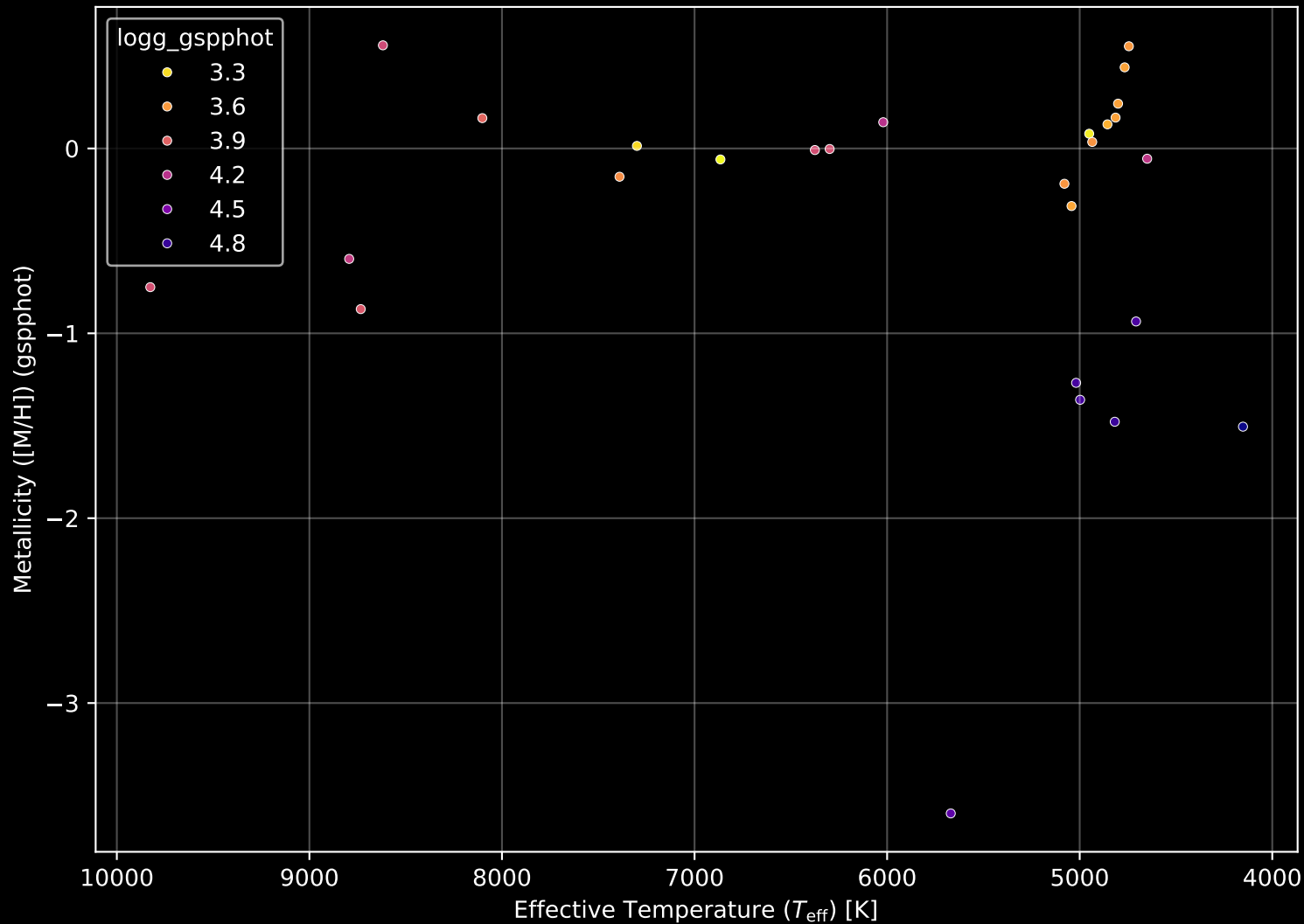
APOGEE DR17 Field: [331+00] Stellar Population Parameters (n= 27)
